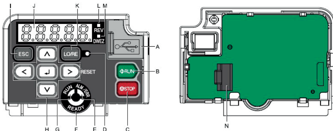
Kuva 1.1 Näppäimistö
